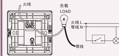
单联单极开关
